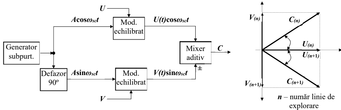
Fig. 2.4. Circuit de modulare a subpurtătoarei de crominanță (sistem PAL): schema bloc și diagrama semnalelor
