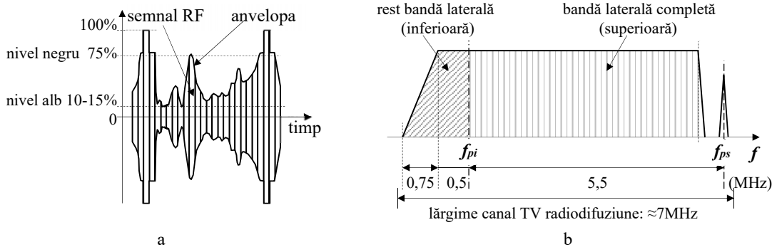
Fig. 2.6. Aspectul semnalului RF modulată în amplitudine cu semnal video complex (a) și ocuparea unui canal TV de radiodifuziune terestră (CCIR PAL-B)
